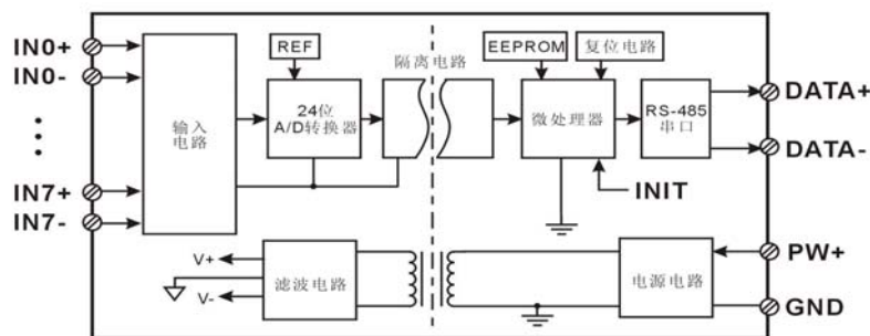
JSD81 内部方框图
